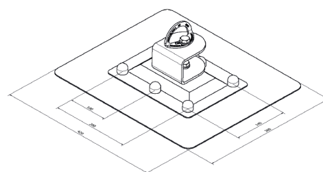
Base disipadora
